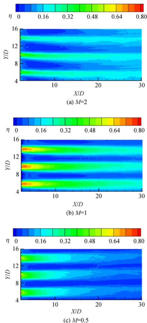
图5 横流条件下不同吹风比冷却效率云图
