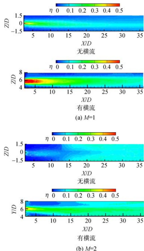
图6 有无横流冷却效率对比
