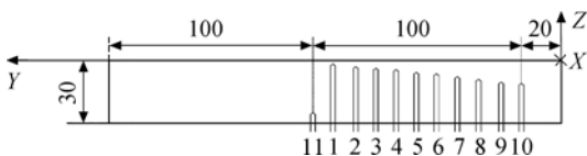
图 3 测量板示意图(单位:mm)
