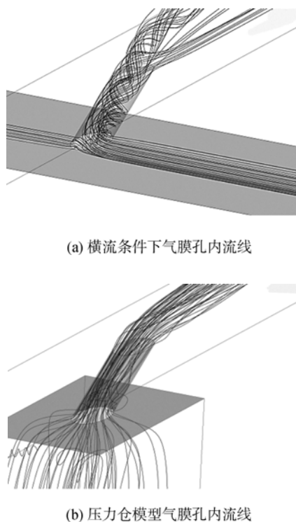
图10 M=1 时气膜孔内流线
