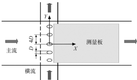
图 2 实验段示意图
