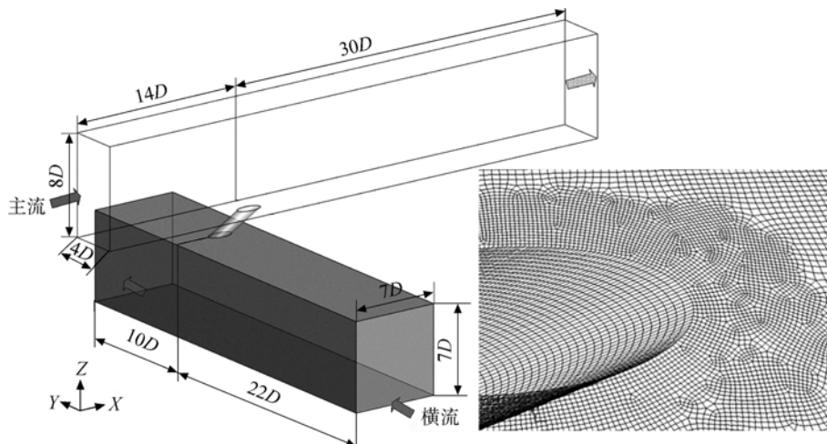
图4 计算模型及网格
