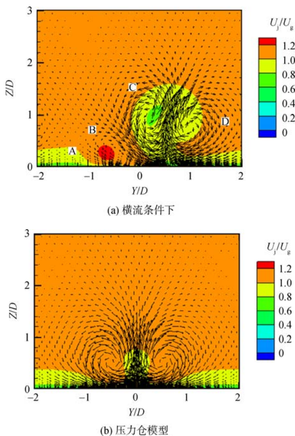
图11 M=1 气膜孔下游截面 X/D=5 处速度矢量云图 Fig. 11 Velocity vector contours at downstream section X/D=5 of film cooling hole for M=1
