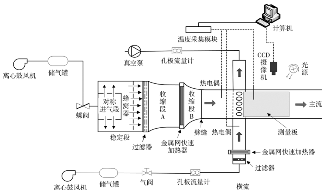
图1 实验系统
